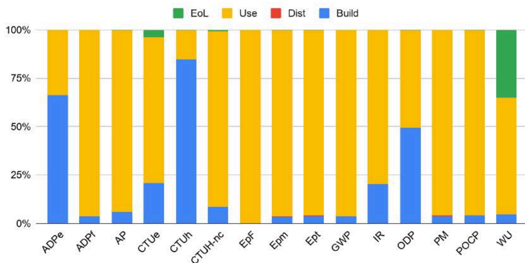
Répartition des impacts par étape du cycle de vie - 2030
