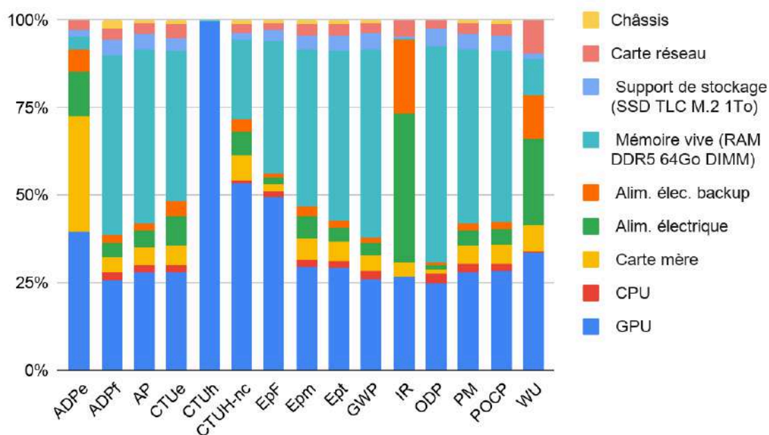
Répartition des composants par impact pour un serveur entrée de gamme
