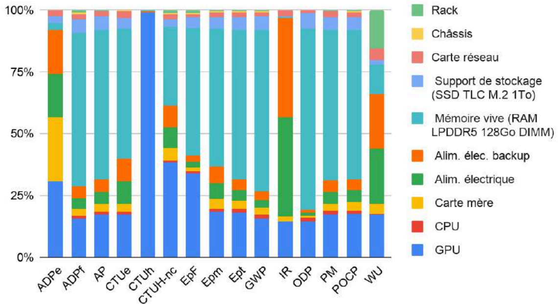
Répartition des composants par impact pour un serveur milieu de gamme
