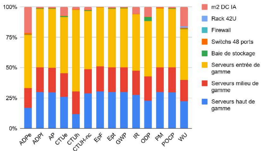
Répartition des impacts par composant - 2030
