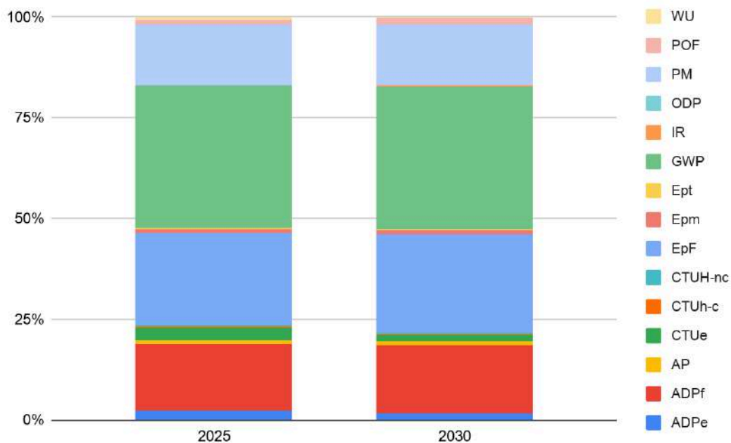
Répartition des impacts en 2025 et 2030
