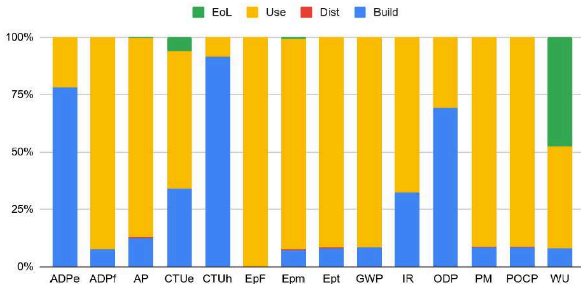
Répartition des impacts par étape du cycle de vie - 2025
