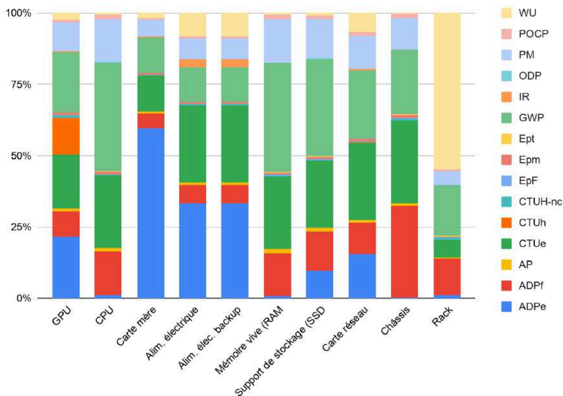
Impacts par composant, serveur milieu de gamme
