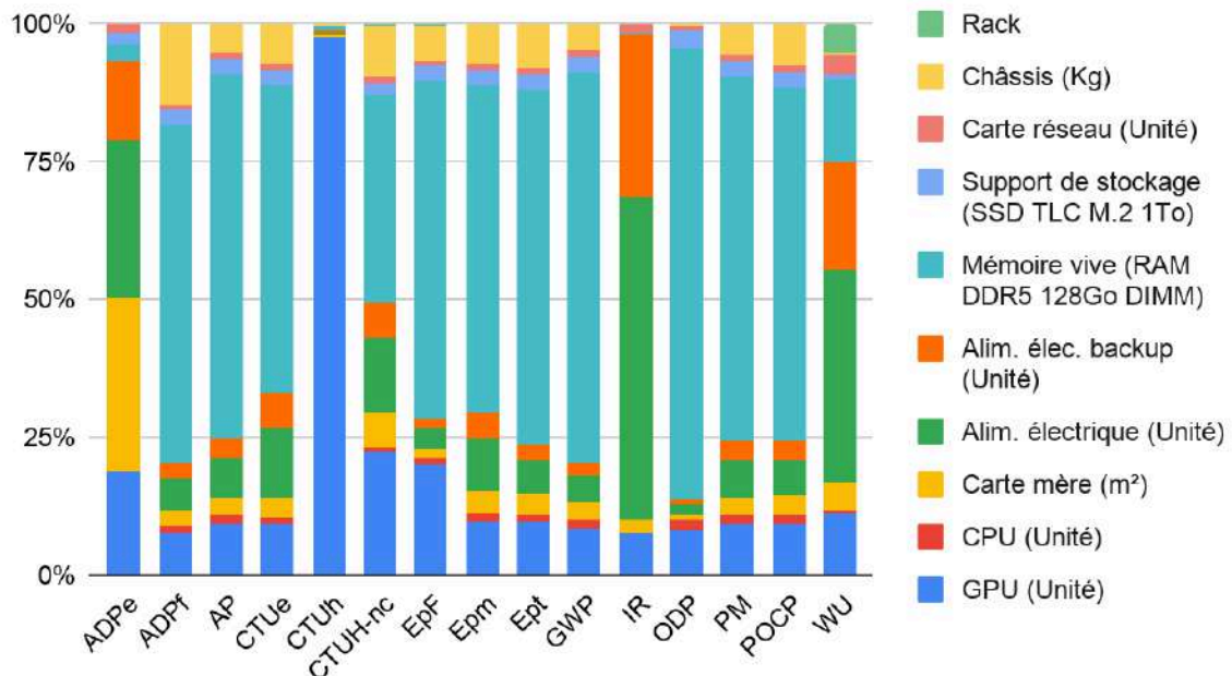
Répartition des composants par impact pour un serveur haut de gamme
