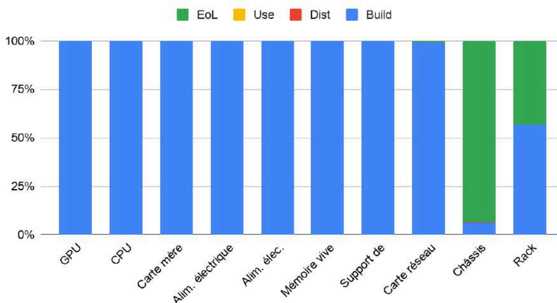
Impacts par étape du cycle de vie pour chaque composant d'un serveur milieu de gamme
